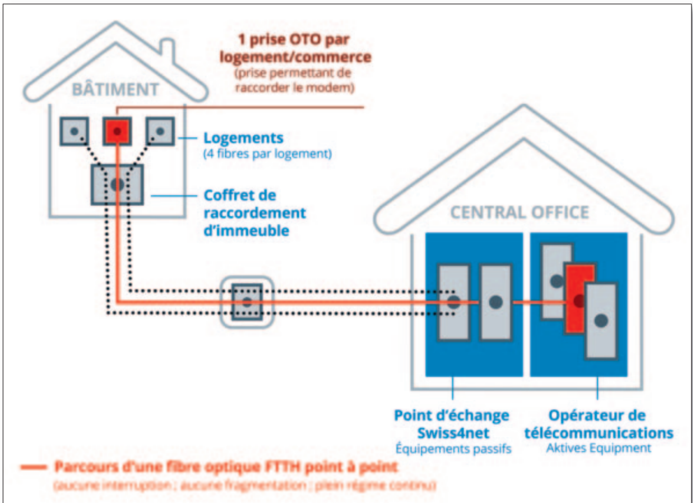
Le réseau en fibre optique FTTH point à point. © swiss4net.ch
